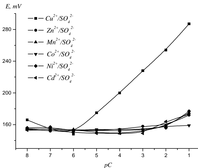
Рис. 2. Вплив сторонніх іонів на відгук купрумселективного електрода (65 % Cu 2 NiTi 3 S 8 та 35 % ДБС)
