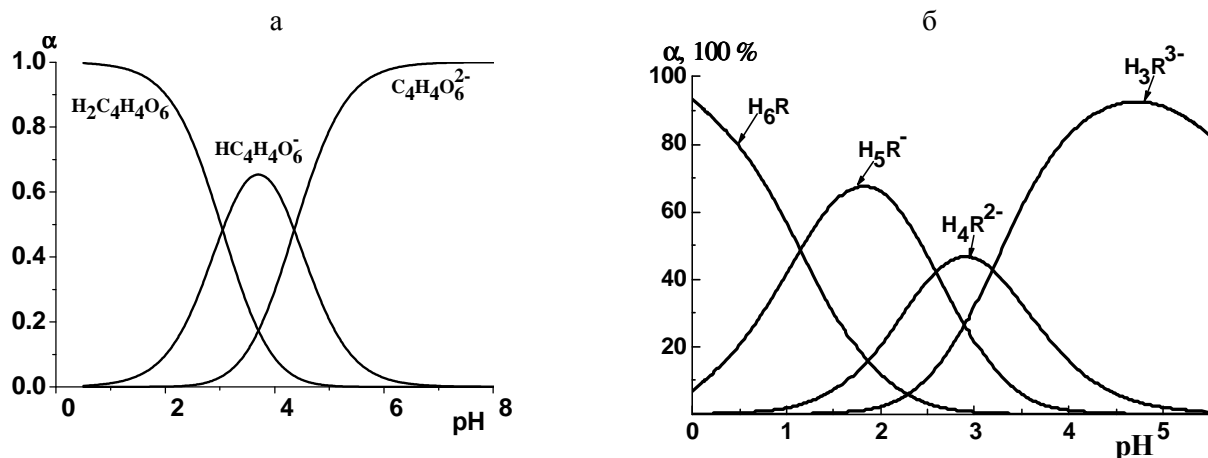
Рис. 4. Розподіл залежно від \text{pH} розчину протолітичних форм КО (а) та протолітичних форм тартратної кислоти (б), константи дисоціації КО: \text{pK}_1 = 1,15 ; \text{pK}_2 = 2,58 ; \text{pK}_3 = 3,23 ; \text{pK}_4 = 6,22 [14] (а) та тартратної кислоти: \text{pK}_1 = 3,04 ; \text{pK}_2 = 4,37 [15] (б)
