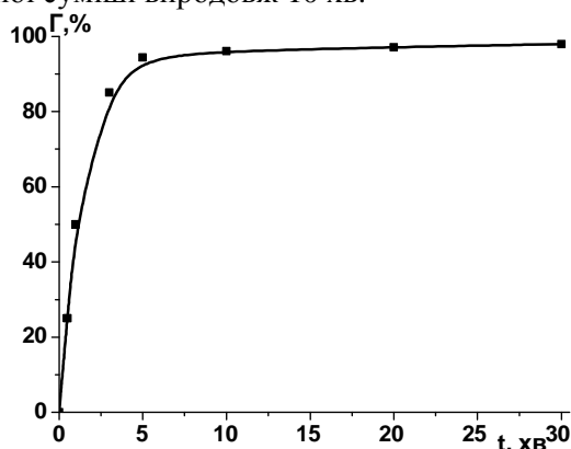
Рис. 1. Залежність сорбції цирконію (IV) модифікованим сорбентом від часу контакту фаз C_{Zr(IV)} = 50 мкмоль/л; рН = 1,6; V/m = 100 мл/г; T = 293 \pm 1 К
