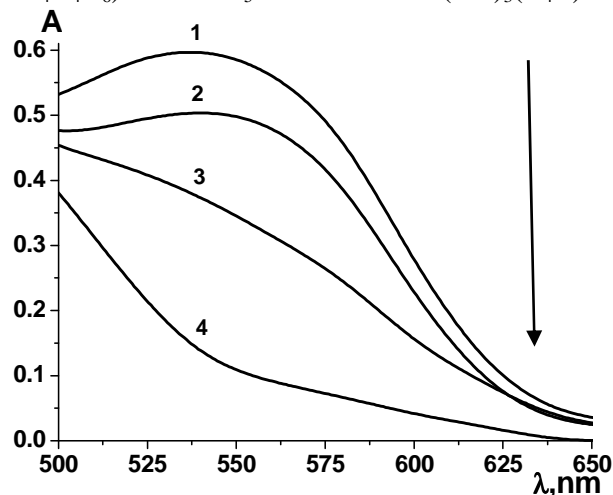
Рис. 3. Спектри поглинання модифікованого сорбенту, обробленого розчином \text{ZrOCl}_2 за відсутності (1) та в присутності тартрату (2–4) a_{\text{КО}} = 3,5 мкмоль/г; \text{pH} = 1,6 ; C_{\text{Zr}} = 50 мкмоль/л; V/m = 200 мг/л; C_{\text{тартрату}} 100 (2); 240 (3); 500 (4) мг/л
