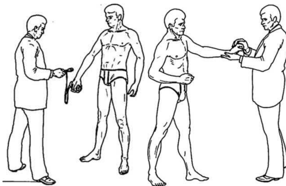
Рис. 3.4.11. Тест Bowden
