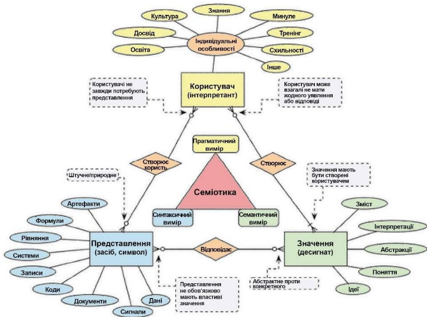
Рис. 5.1. Діаграма сутність-зв'язок, що відображає поняття семіотики [73]
