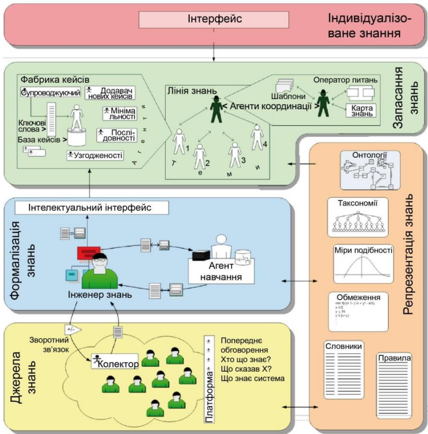
Рис. 5.5. Архітектура колаборативної мультиекспертної системи, орієнтованої на забезпечення продуктової лінії 76
