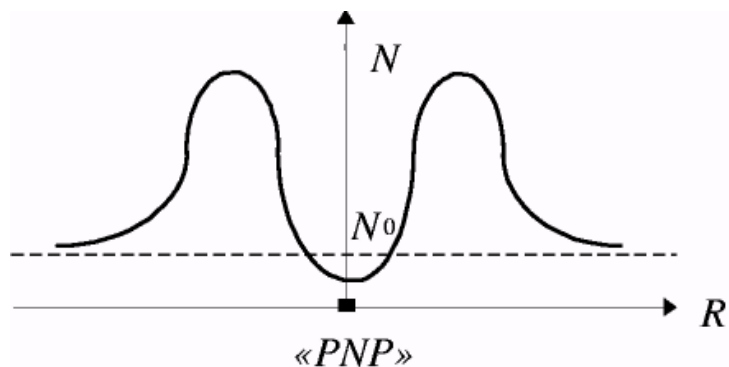
Рис. 6 Залежність рівня модуляційних шумів 2-ий гармоніки напівпровідникового рп-переходу від відстані від об'єкта до осі антеною системи локатора: «PNP» - точка розташування напівпровідникового елемента; N - рівень шуму в головних телефонах; N0 - рівень шуму в головних телефонах при відсутності нелінійного перевідбиваючого об'єкта; R - відстань від точки розташування перевідбиваючого об'єкта до осі антенної системи пристрою.
