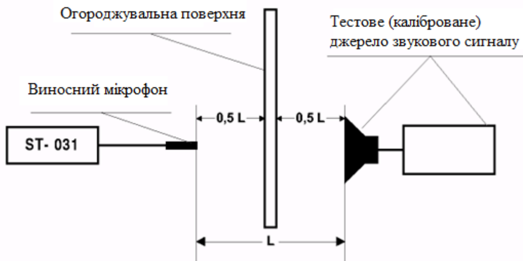
Рис. 9. Схема оцінки звукоізоляції приміщень
