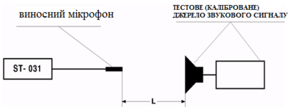
Рис.8. Схема калібрування індикаторів рівня звукового сигналу приладу ST-031
