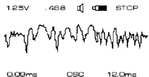
Рис.5. Осцилограма цифрового сигналу передачі мовної інформації у дротовій лінії (той самий сигнал)
