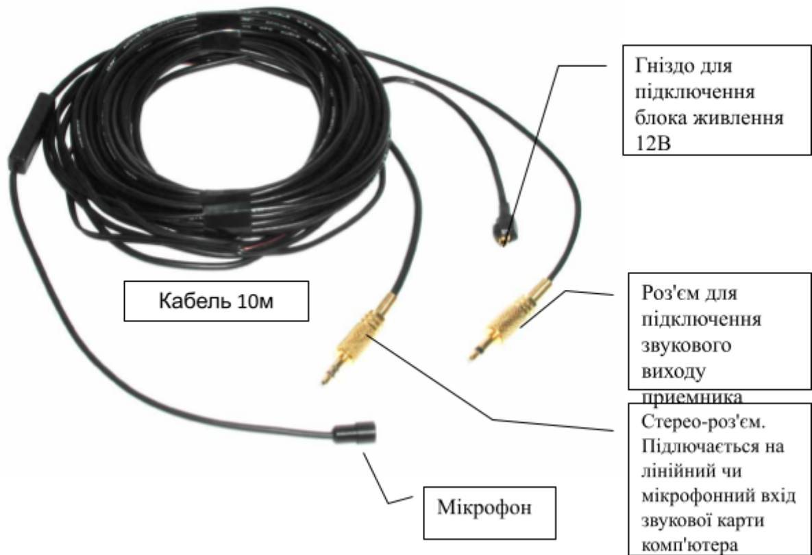
Рис. 1. Кабель з виносним мікрофоном.
