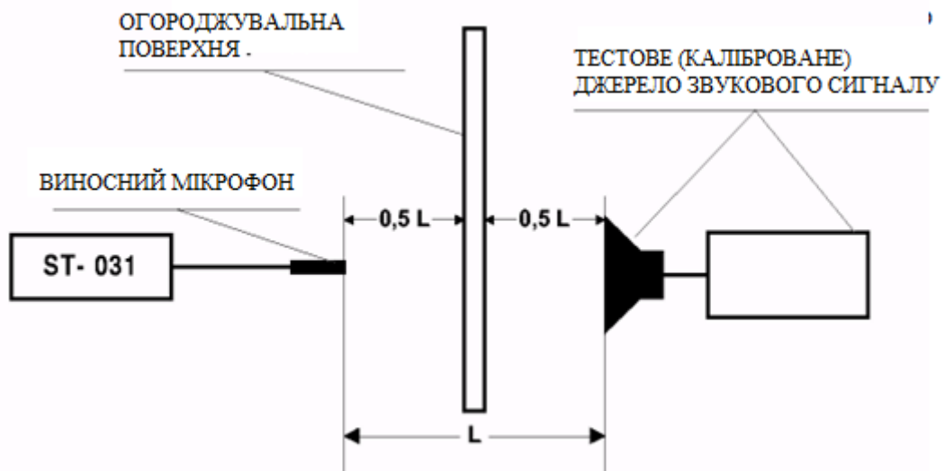
Рис. 8. Схема оцінки звукоізоляції приміщень
