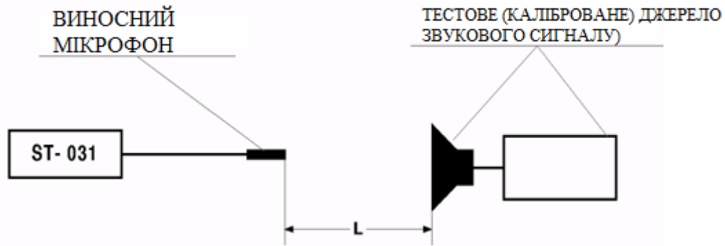
Рис. 7. Схема калібрування індикаторів рівня звукового сигналу приладу ST 031
