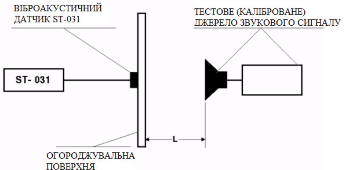
Рис. 6. Схеми оцінки віброакустичних властивостей і віброакустичного захисту приміщень
