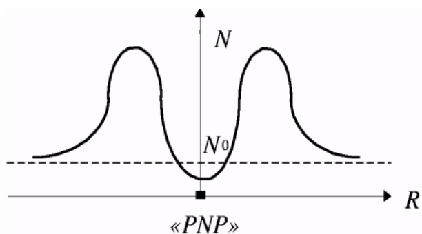
Рис. 4. Залежність рівня
