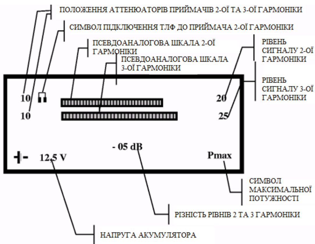
Рис. 2. Вид інформації, що відображається, на дисплеї
