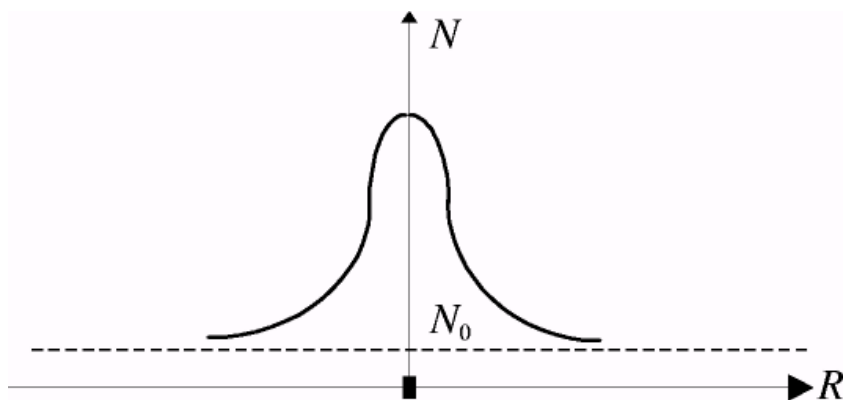
Рис. 5 Залежність рівня модуляційних шумів 2-ий гармоніки корозійного рп-переходу від відстані від об'єкта до осі антенною системи локатора: «К» - точка розташування корозійного рп - переходу; N - рівень шуму в головних телефонах; N_0 - рівень шуму в головних телефонах за відсутності нелінійного перевідбиваючого об'єкта; R - відстань від точки розташування перевідбиваючого об'єкта до осі антенної системи пристрою.
