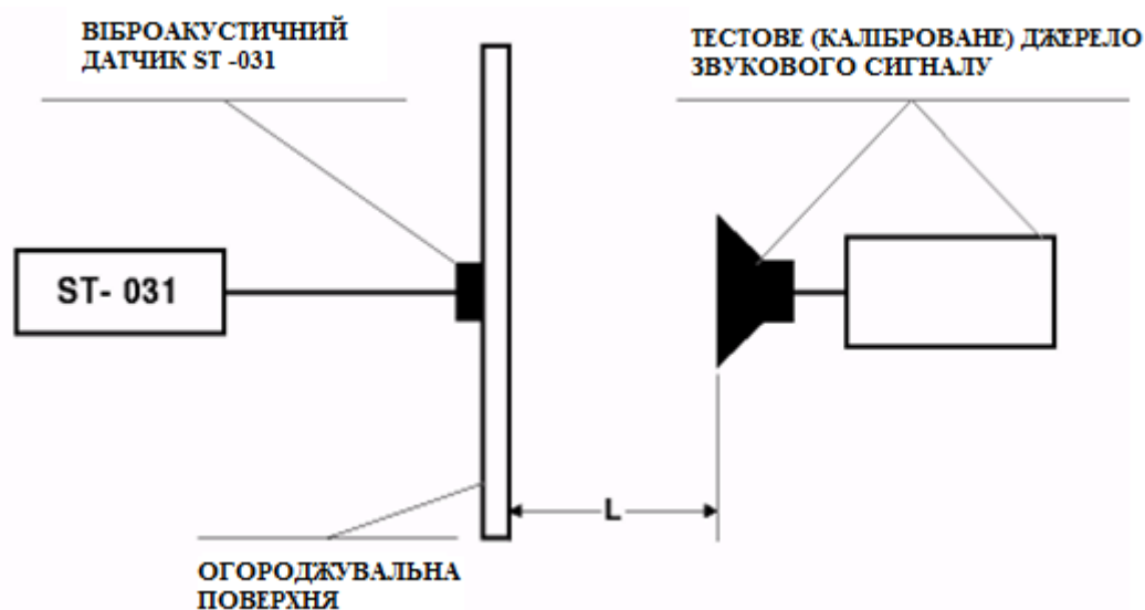
Рис. 7. Схема оцінки віброакустичних властивостей і віброакустичного захисту приміщень
