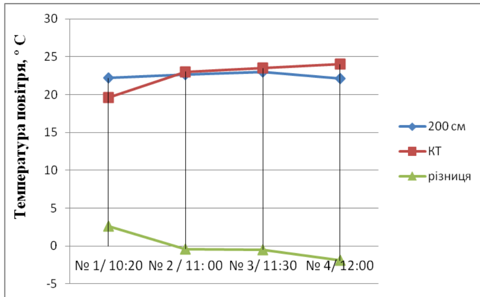
Рис. 2.2.3. Відхилення температури повітря на висоті 200 см від поверхні ґрунту на точках маршруту: майдан Президента Грушевського – «Адреналін Сіті» (04.07.17 р.) порівняно з контрольною точкою
