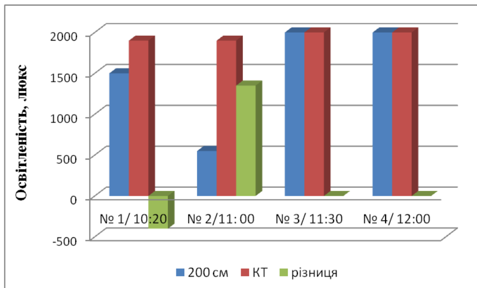
Рис. 2.2.8. Відхилення освітленості території на висоті 200 см від поверхні ґрунту на точках маршруту: майдан Президента Грушевського – «Адреналін Сіті» (04.07.17 р.) порівняно з контрольною точкою
