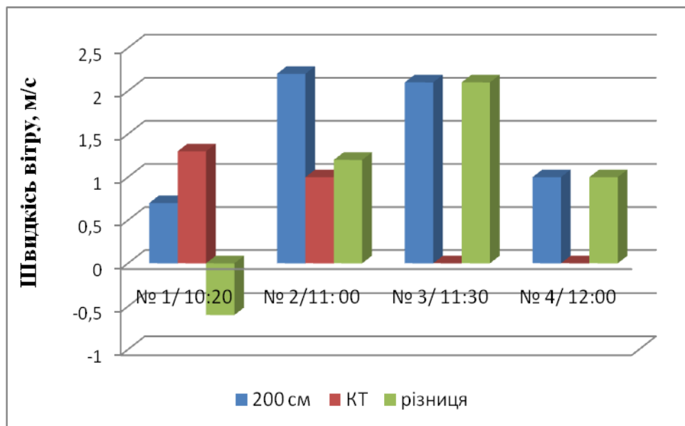
Рис. 2.2.10. Відхилення швидкості вітру на точках маршруту: майдан Президента Грушевського – «Адреналін Сіті» (04.07.17 р.) порівняно з контрольною точкою
