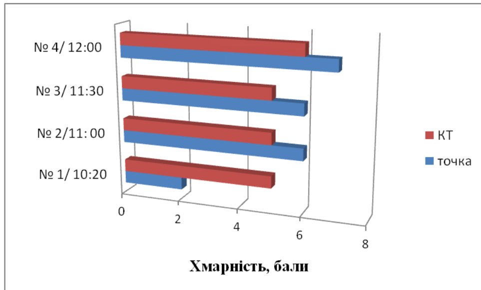
Рис. 2.2.9. Мінливість в стані неба на точках маршруту: майдан Президента Грушевського – «Адреналін Сіті» (04.07.17 р.) порівняно з контрольною точкою
