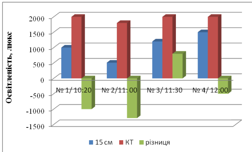
Рис. 2.2.7. Відхилення освітленості території на висоті 15 см від поверхні ґрунту на точках маршруту: майдан Президента Грушевського – «Адреналін Сіті» (04.07.17 р.) порівняно з контрольною точкою
