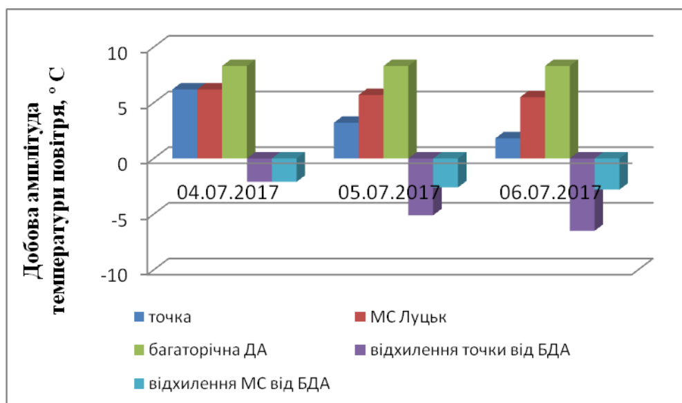
Рис. 2.1.6. Відхилення добової амплітуди температури повітря точки спостереження на висоті 200 см, метеостанції Луцьк від середньої багаторічної добової амплітуди з 04.07 - 06.07.2017 р.
