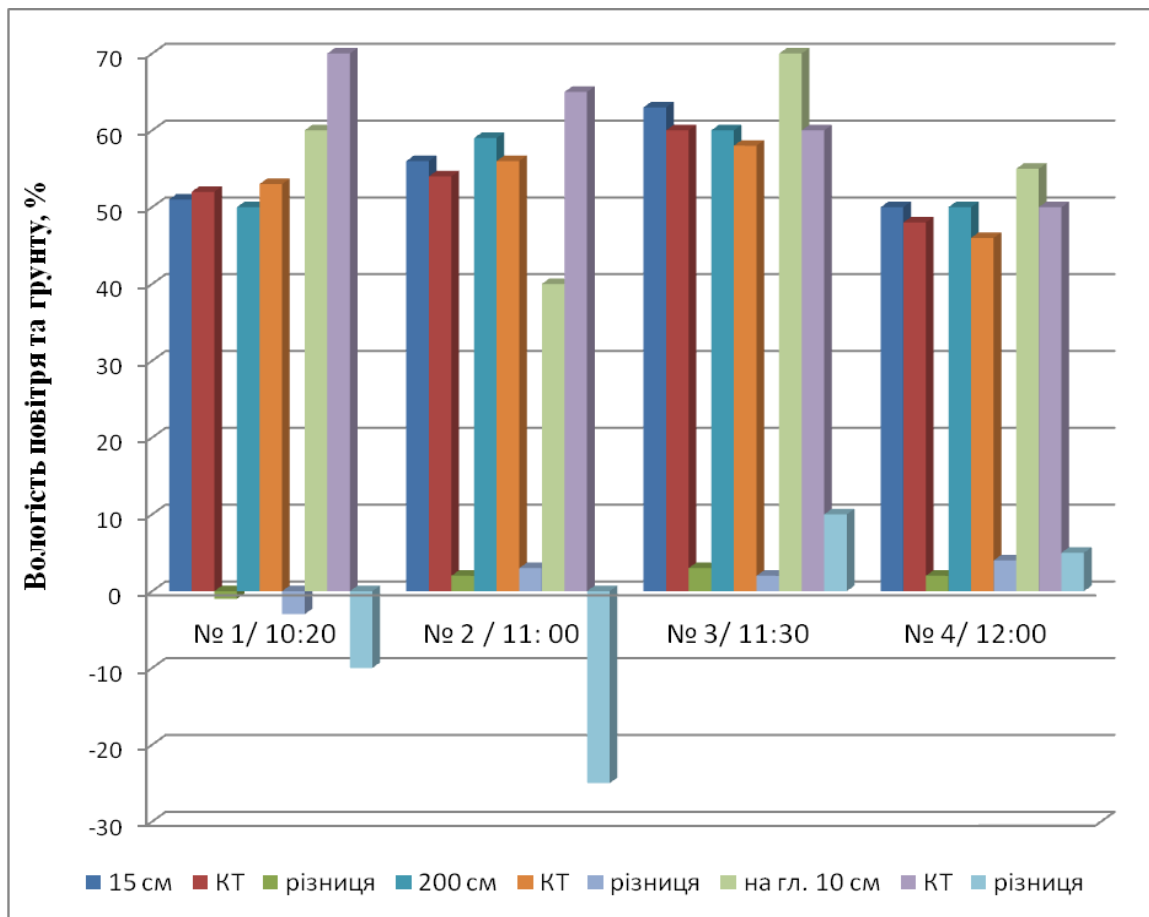
Рис. 2.2.5. Мікрокліматична мінливість вологості повітря і ґрунту на точках маршруту: майдан Президента Грушевського – «Адреналін Сіті» (04.07.17 р.) та їх відхилення порівняно з контрольною точкою
