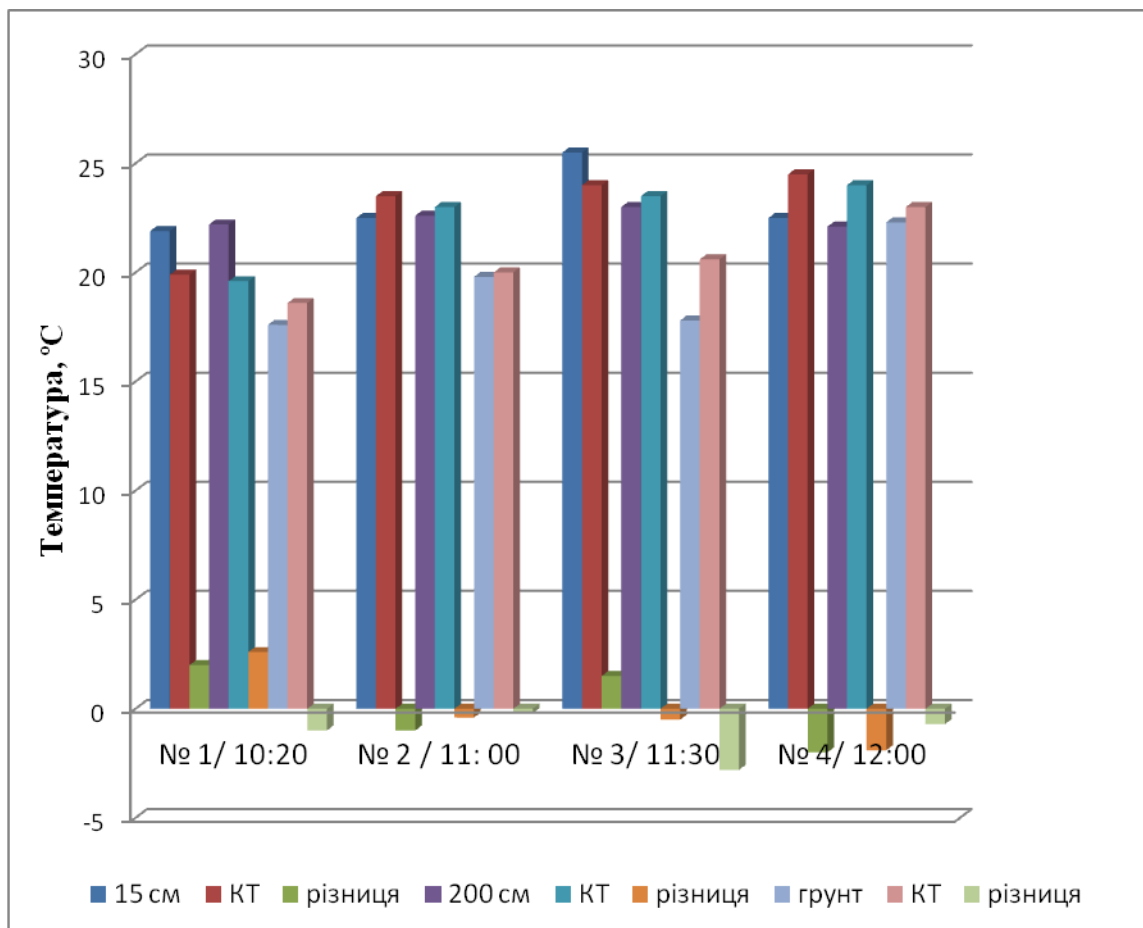
Рис. 2.2.1. Мікрокліматична мінливість температури повітря і ґрунту на точках маршруту: майдан Президента Грушевського – «Адреналін Сіті» (04.07.17 р.) та їх відхилення порівняно з контрольною точкою
