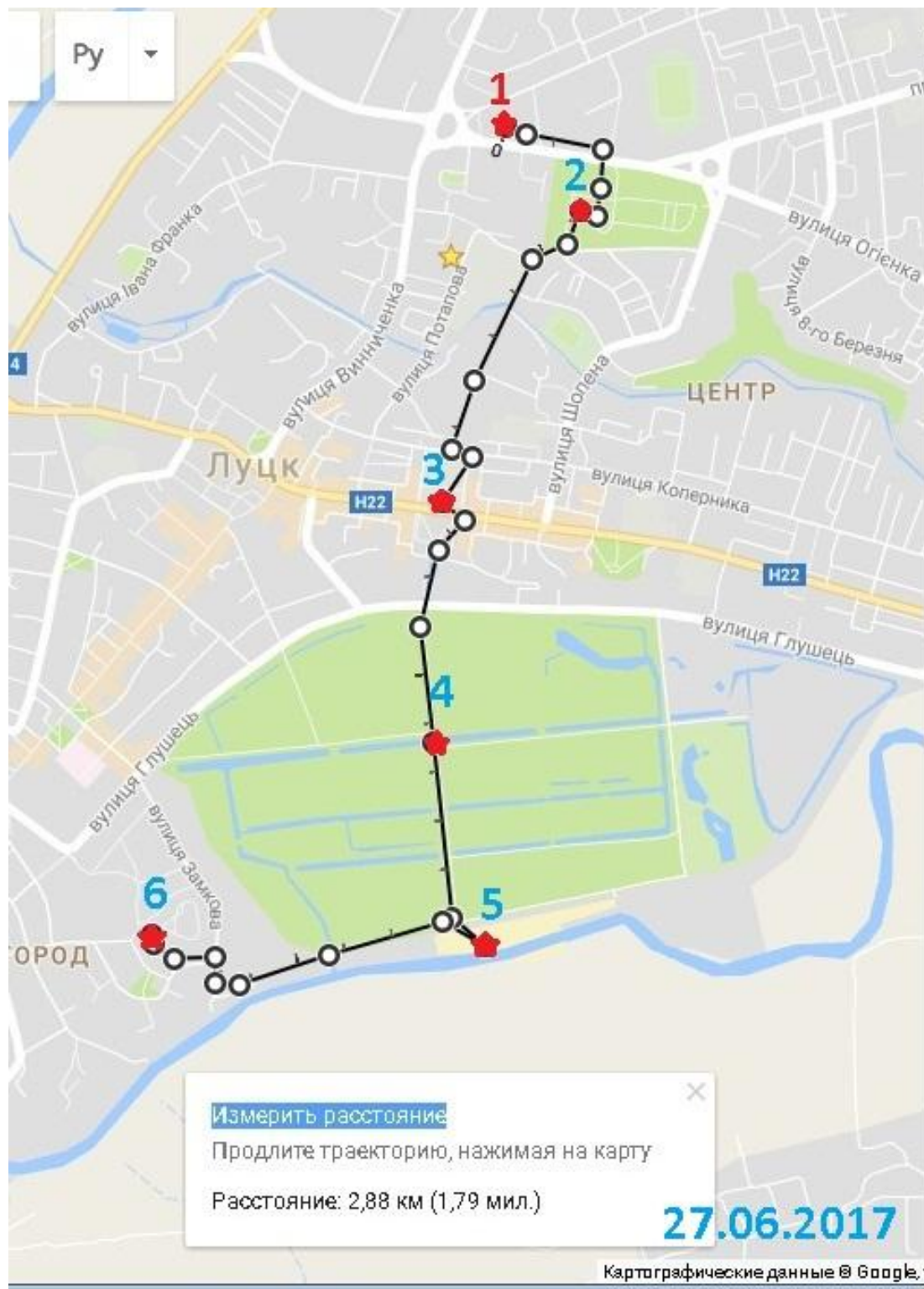
Рис. 2.2.1. Приклад розробленого мікрокліматичного маршруту за допомогою інструментів картографічних даних Google: майдан Президента Грушевського – Замок Любарта
