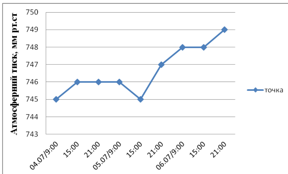
Рис. 2.1.11. Денний хід атмосферного тиску точки спостереження з 04.07 - 06.07.2017 р.
