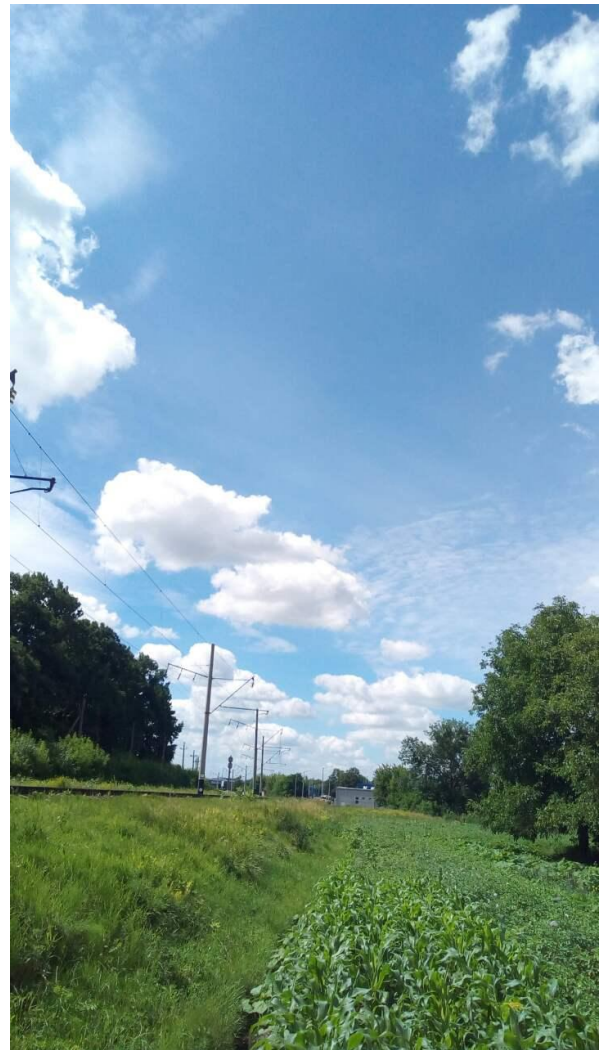
Фото 2.2.1. Купчасті середні – Cumulus mediocris (4.07.17 – 12:00)
