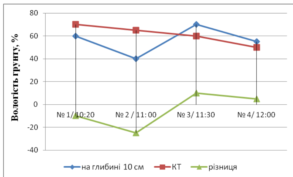
Рис. 2.2.5. Мікрокліматична мінливість вологості повітря і ґрунту на точках маршруту: майдан Президента Грушевського – «Адреналін Сіті» (04.07.17 р.) та їх відхилення порівняно з контрольною точкою
