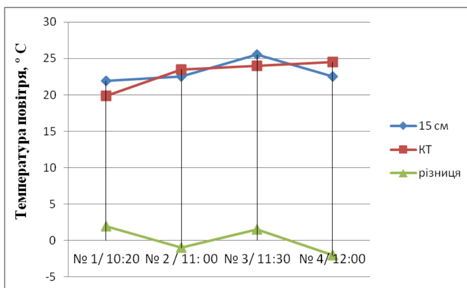
Рис. 2.2.2. Відхилення температури повітря на висоті 15 см від поверхні ґрунту на точках маршруту: майдан Президента Грушевського – «Адреналін Сіті» (04.07.17 р.) порівняно з контрольною точкою
