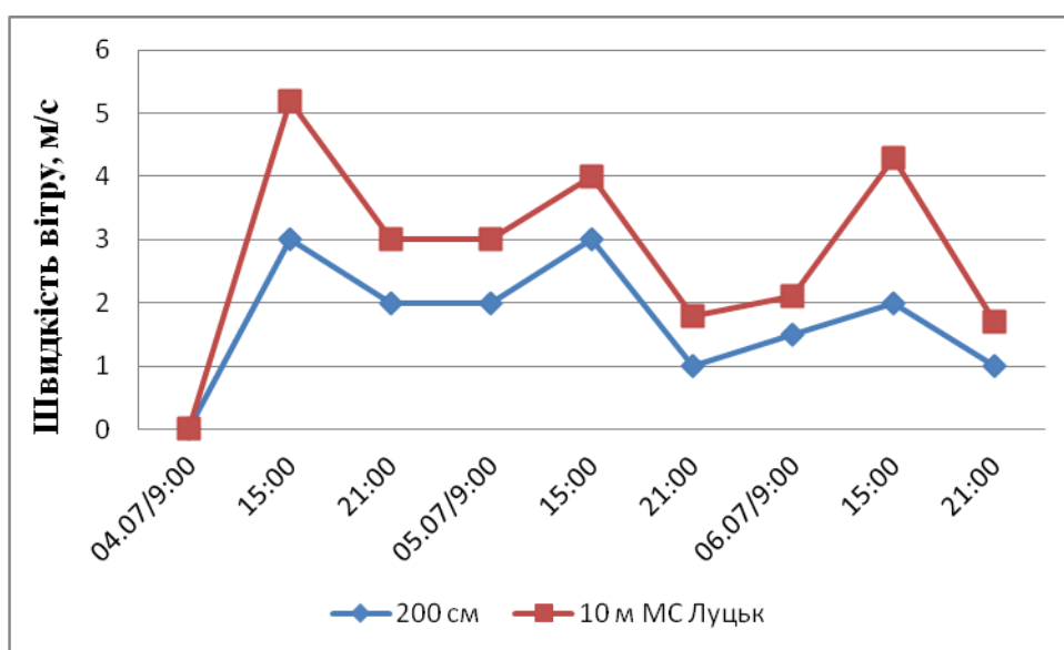
Рис. 2.1.12. Денний хід швидкості вітру точки спостереження на висоті 200 см і 10 м на метеостанції Луцьк з 04.07 - 06.07.2017 р.
