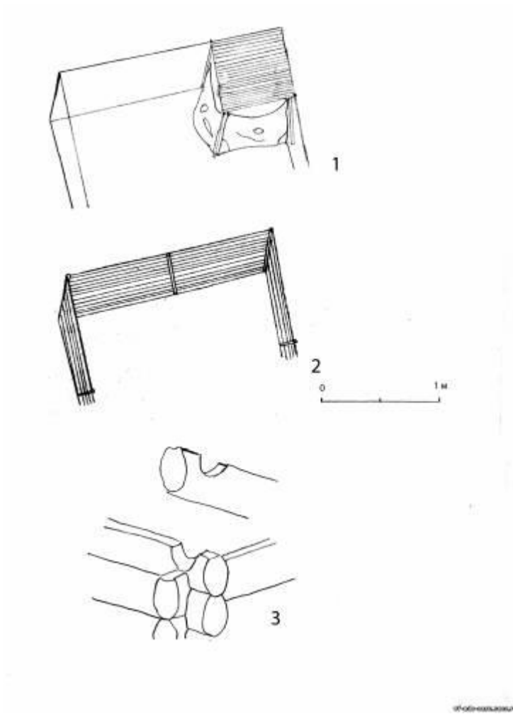
Рис.1. Основні елементи, використані в реконструкції житла з Богушівки: 1 – розміщення пічки та навісу над неї у реконструкції; 2 – дерев'яний каркас стін; 3 - кріплення колод у реконструкції
